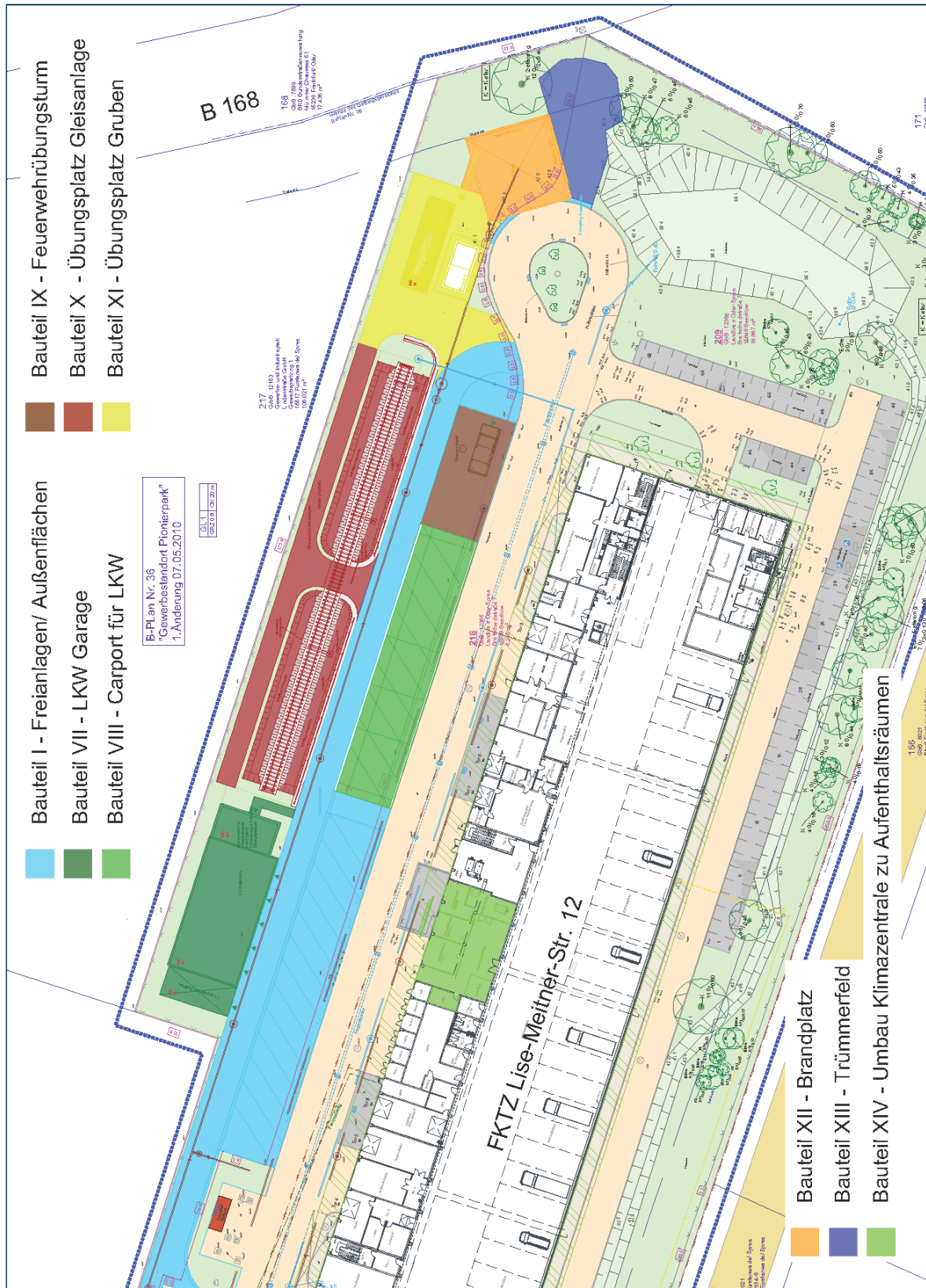
Lageplan - Ausschnitt 2
