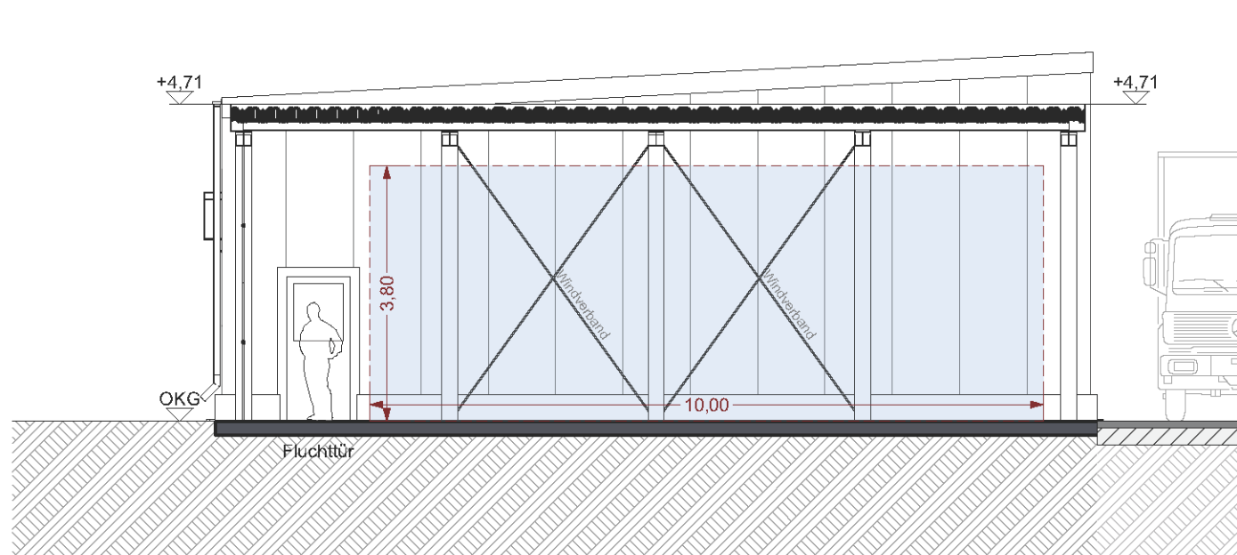
EP_SN-03 Schnitt Außenstellplatz 1:100
