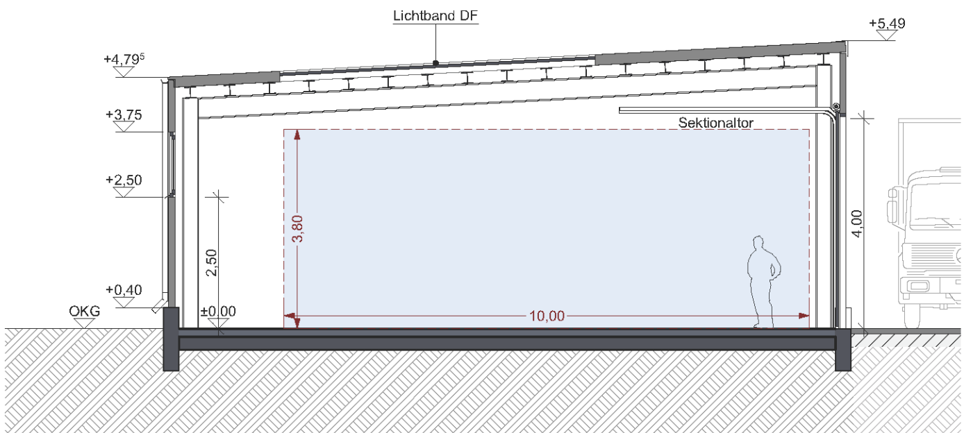
EP_SN-01 Schnitt Querschnitt LKW Garage 1:100
