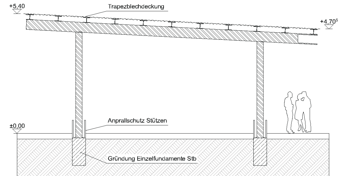
EP_SN-02 Schnitt parallel zur Tragkonstruktion 1:100
