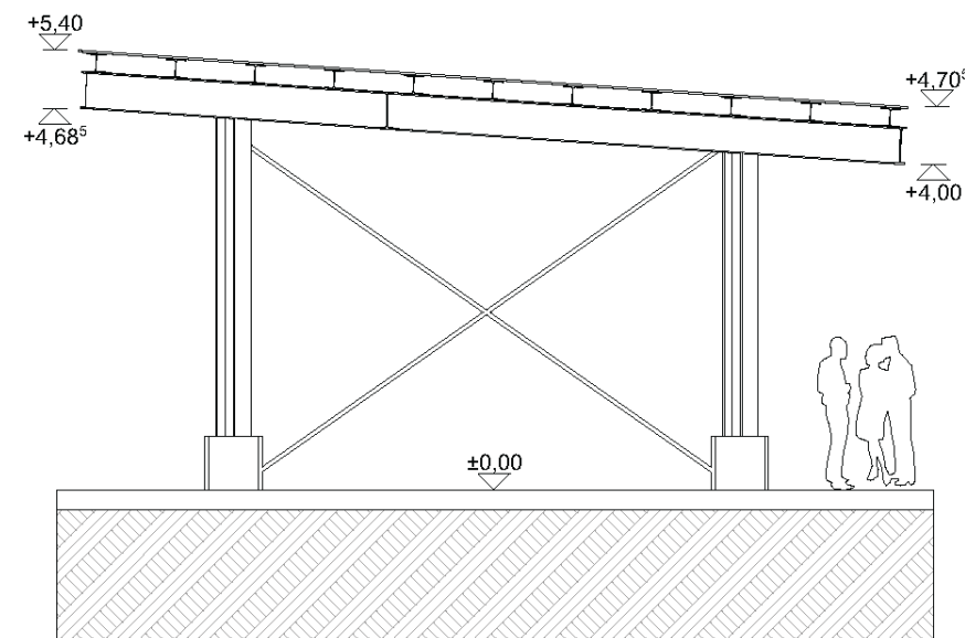
EP_SN-01 Schnitt Querschchnitt 1:100
