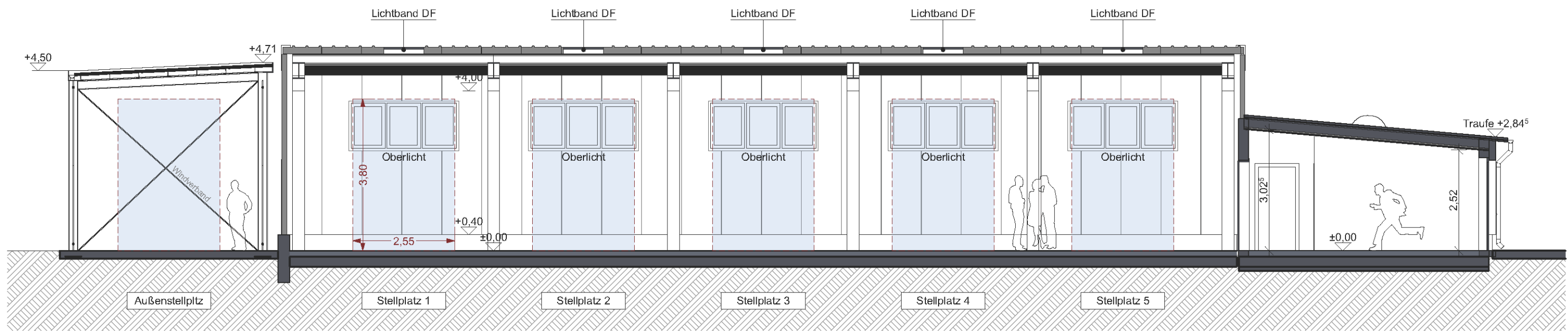
EP_SN-02 Schnitt Längs 1:100
