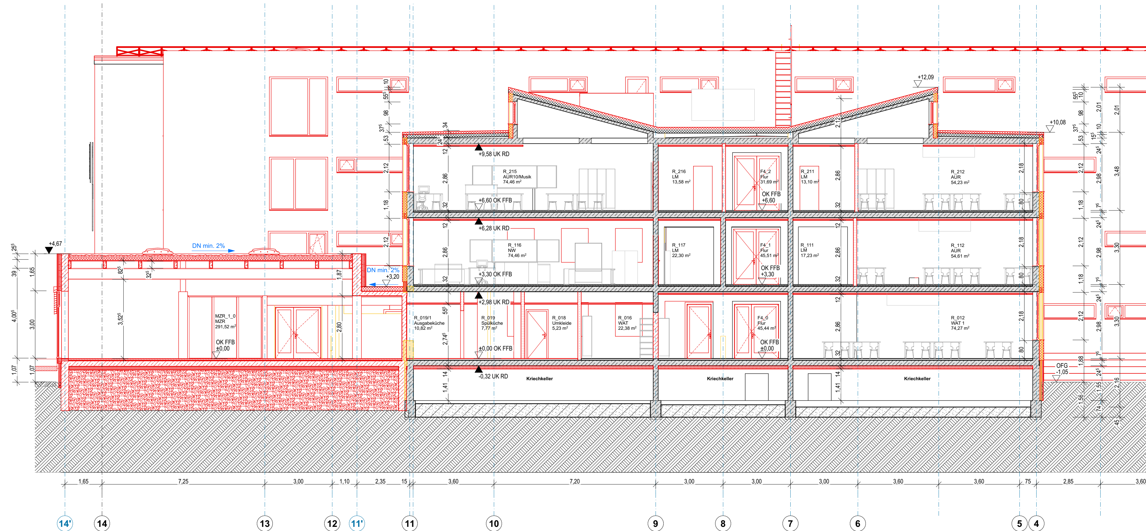
Schnitt E-E
